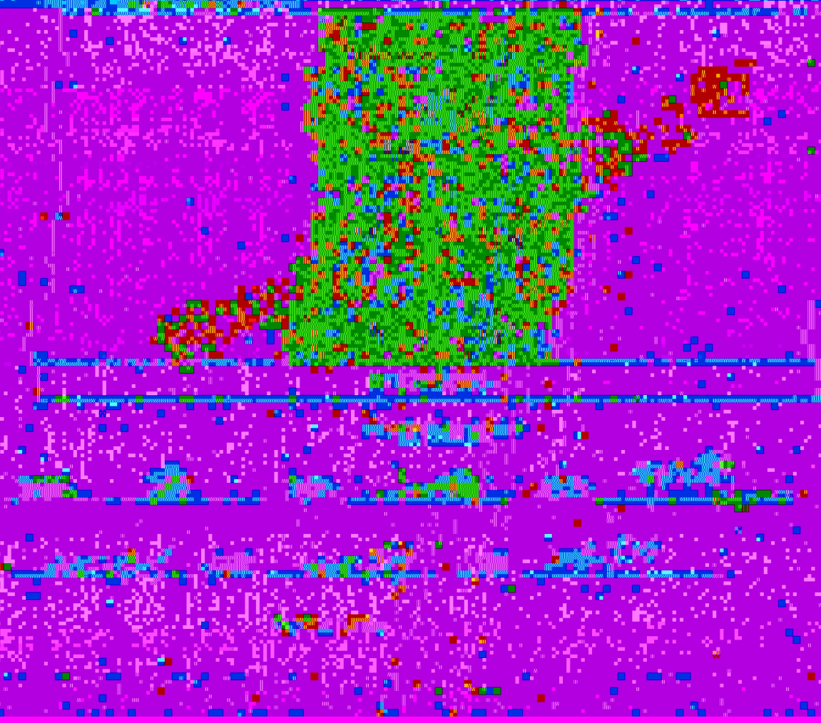
图 11-1 样品谱图
